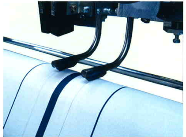
切断面を熱溶着している図 (HT-1L) Melt-down the fabric by L type heater (HT-1L)
